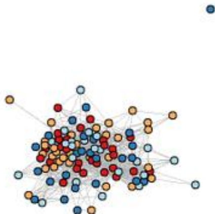
ActionPropertyTool
